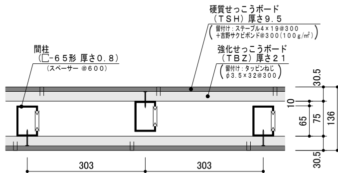
水平断面図
